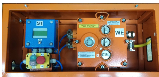
Układ kontroli i zasilania prasy wulkanizacyjnej
