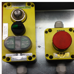
Przyciski sterownicze zamontowane w osłonie
